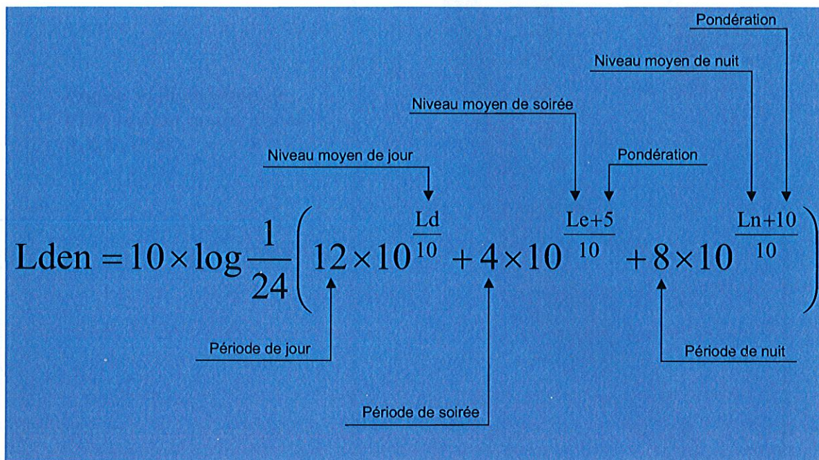
Figure 2 : Indice L_{den} : formule de pondération du bruit.
